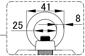
アイナット部拡大図 尺度(2/5)
