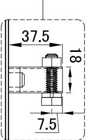
インタージエントホルダー一部拡大図 尺度(2/5)
