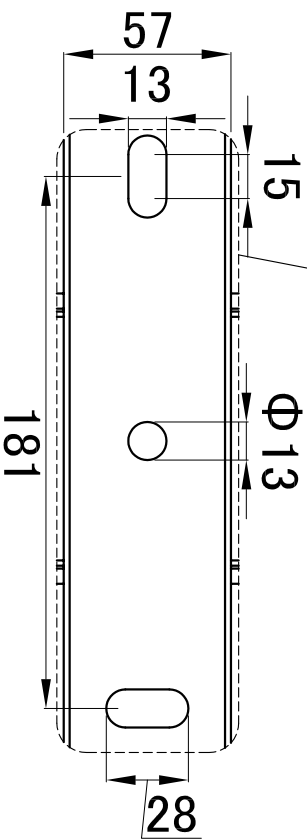
金具取付穴部拡大図
