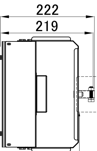
インテリジェントホルダー取付要領図
