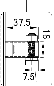
インテリジェントホルダー一部拡大図 尺度(2/5)
