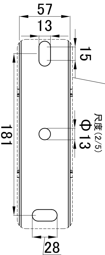
金具取付穴部拡大図
